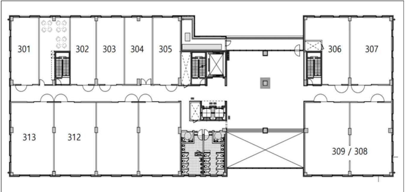
지상3층 평면도 - 층고 3.9m
