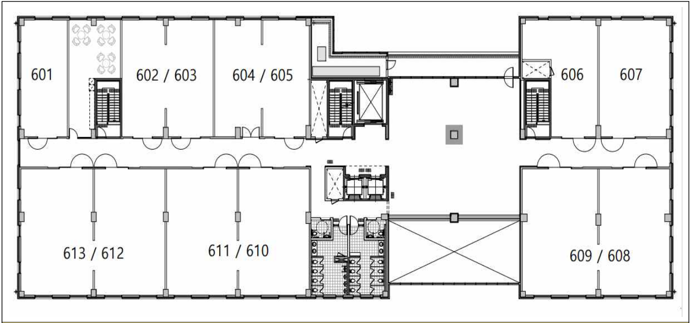
지상6층 평면도 - 층고 3.9m
