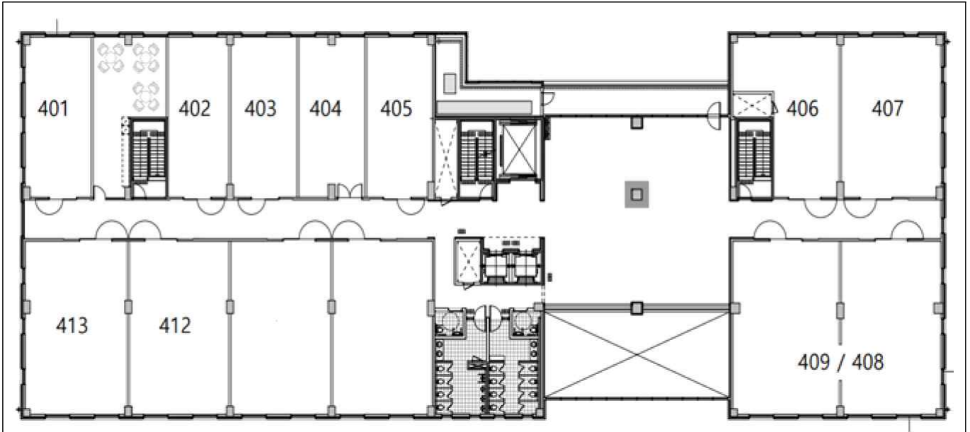
지상4층 평면도 - 층고 3.9m
